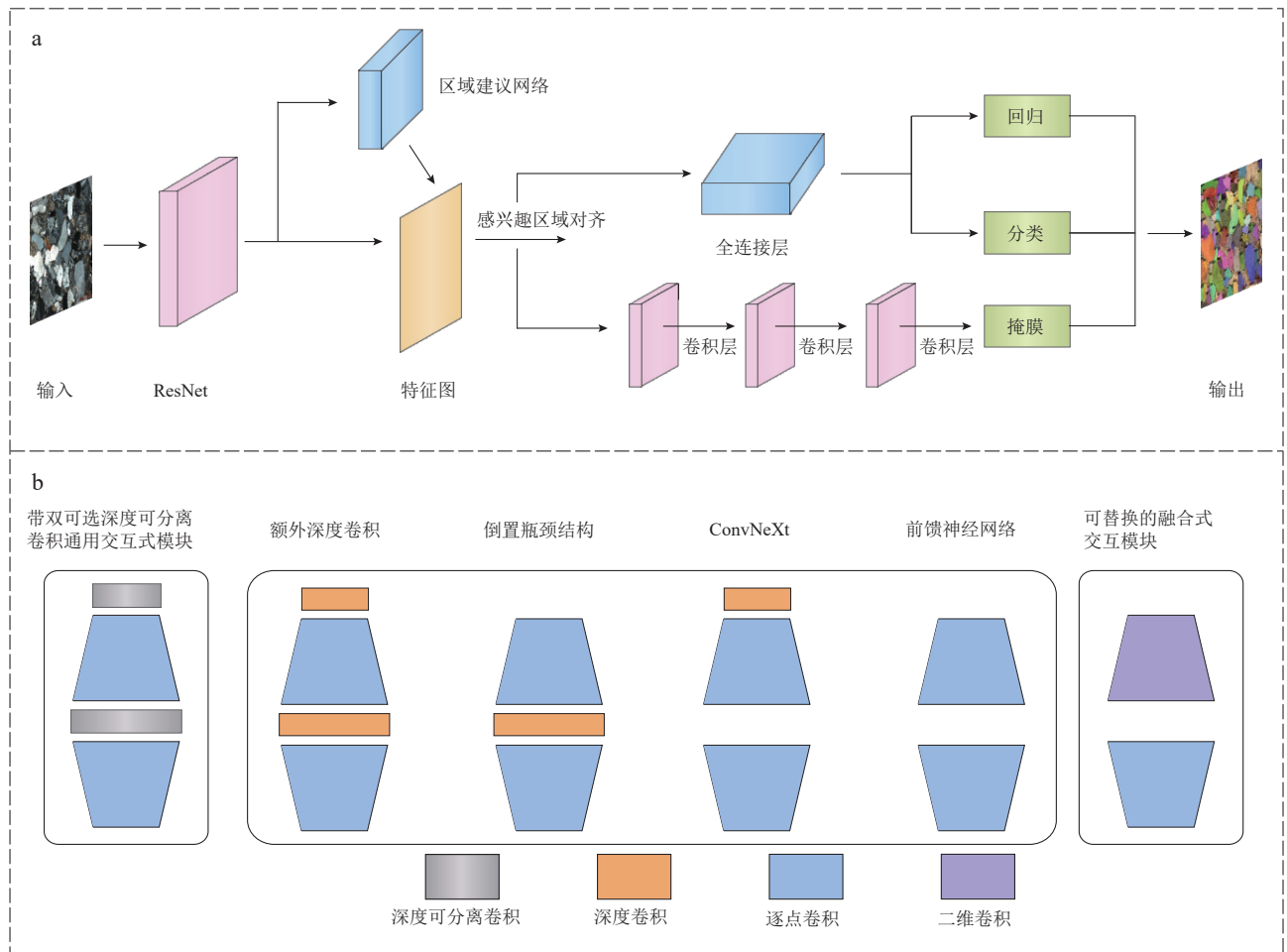
图3 改进的砂岩图像分割与分类深度学习模型结构示意图
