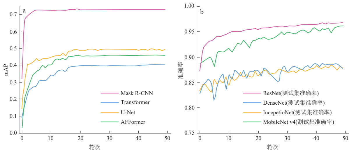
图4 各深度学习模型性能随训练轮次变化曲线
