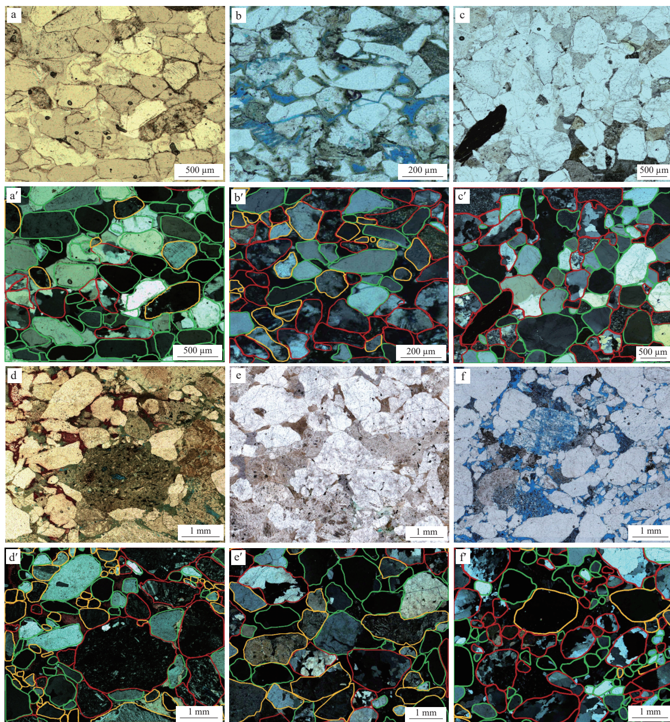
图5 不同盆地6个砂岩样品代表性视域的深度学习分析结果
