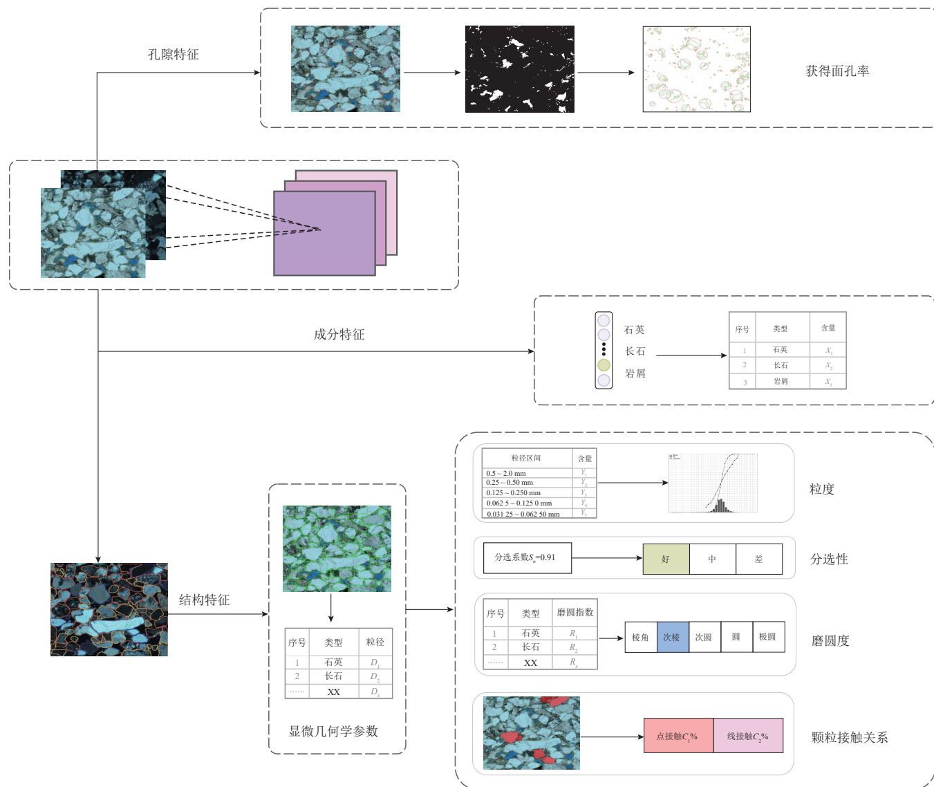
图6 鄂尔多斯盆地东南部上三叠统延长组S2样品岩相学特征定量提取结果图
